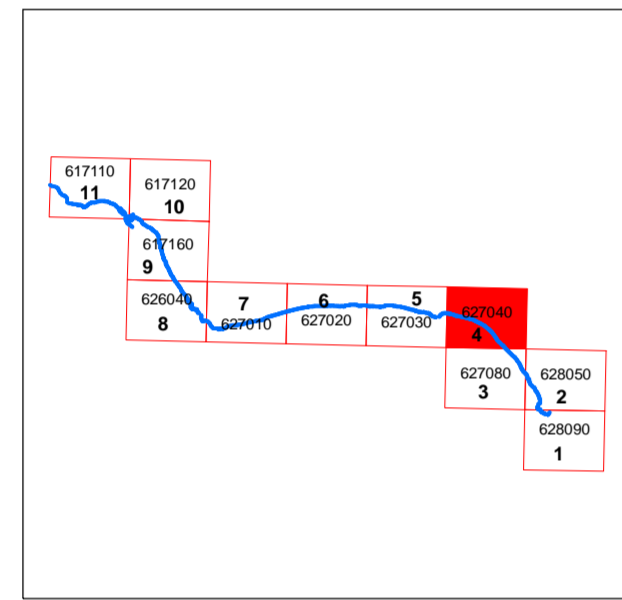
Carta della tipologia costiera e dell'evoluzione delle linee di riva N°4 Scala 1:5.000
